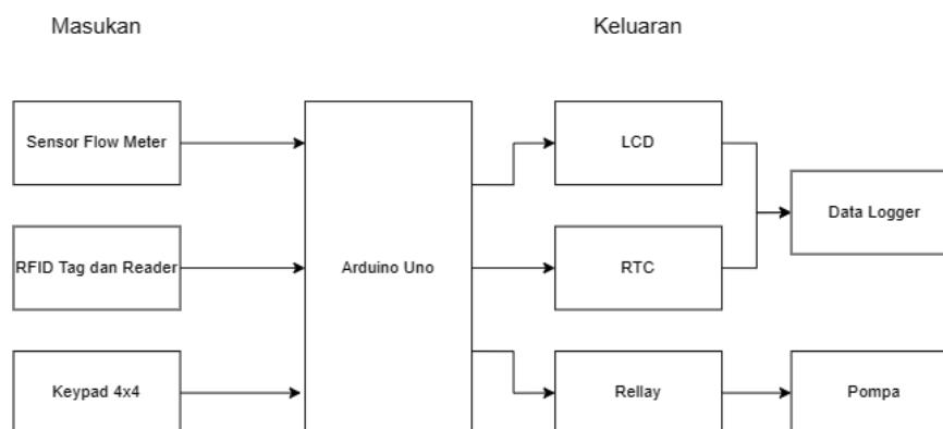
Gambar 1. Konsep Blok Sistem
