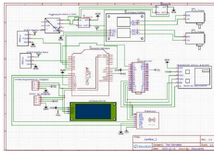
Gambar 5. Desain Perancangan Hardware
