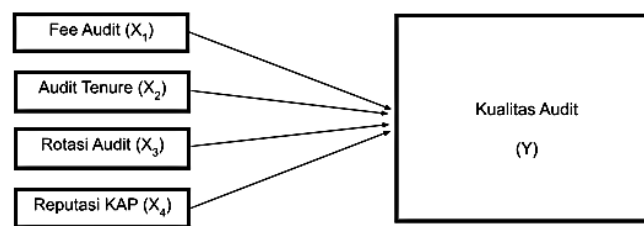
Gambar 1. Kerangka Konseptual
